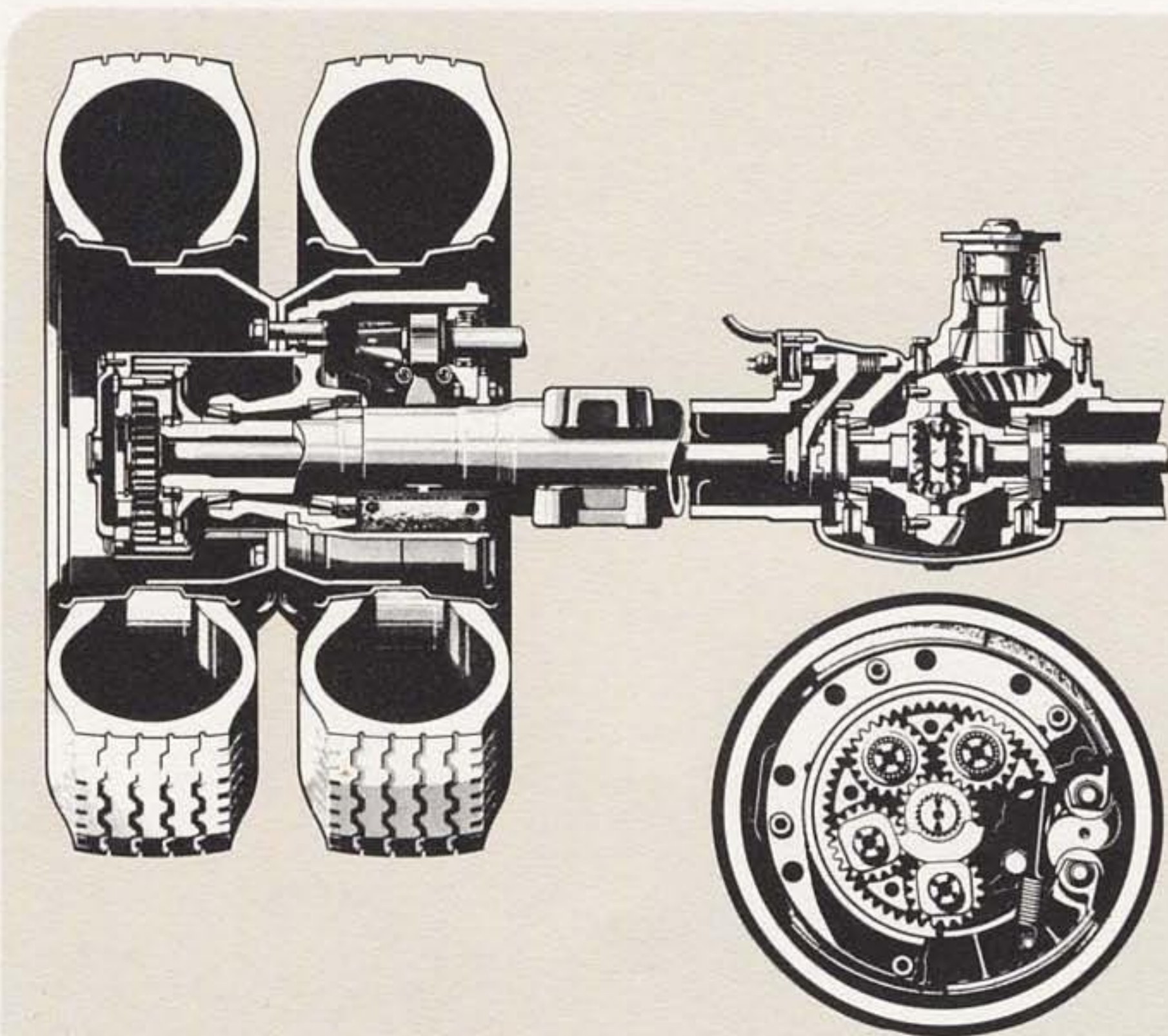
Het zonnewiel van de in de naaf gemonteerde reductie drijft vijf planeetwielen aan. Hier vindt de belangrijkste reductie plaats en wordt het hoge koppel ontwikkeld.
