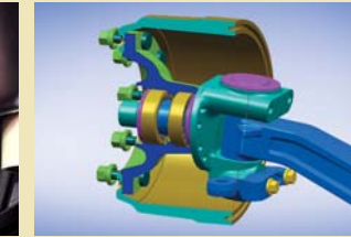
신형 조향축
